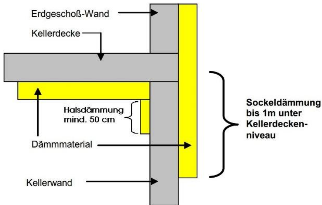
Abbildung: Halsdämmung (NÖ Energie- und Umweltagentur GmbH)
